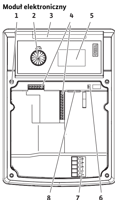
Rys. 9: Moduł elektroniczny
