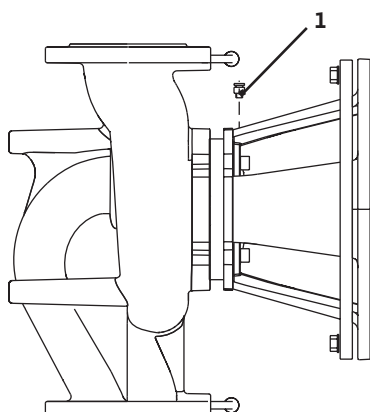
Rys. 35: Zawór odpowietrzający
