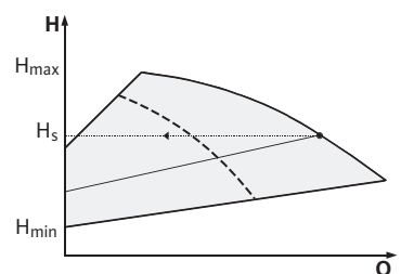
Rys. 15: Regulacja \Delta p -v (praca równoległa)
