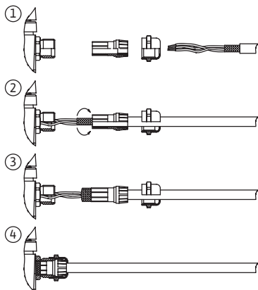
Rys. 19: Ekranowanie przewodów
