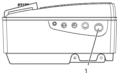
Rys. 18: Kablowe złącze śrubowe M25
