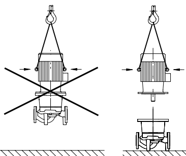
Rys. 16: Podwieszanie silnika
