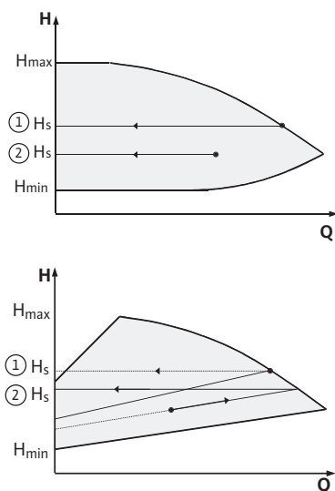
Rys. 37: Regulacja \Delta p\text{-}c/\Delta p\text{-}v
