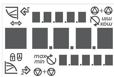
Rys. 25: Test wyświetlacza
