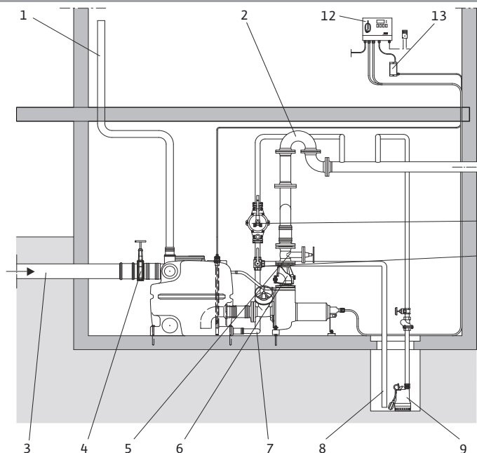
Rys. 9: Przykład instalacji
