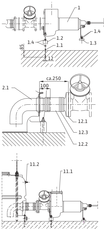
Rys. 4: Ustawienie pomp
